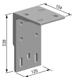
Plafondbevestiging (L)
