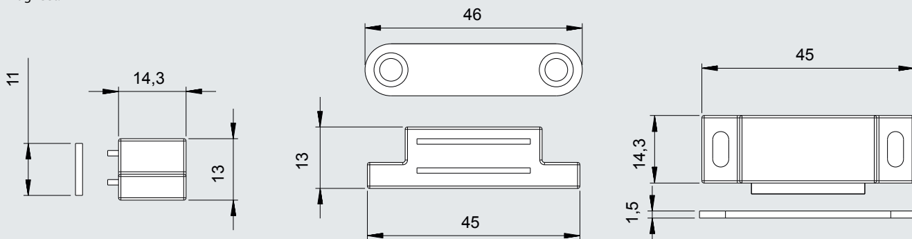
Magneet:
