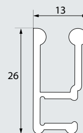
Glijrail:
