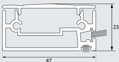
Doorsnede:
