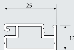
Doorsnede:
