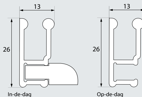
Doorsnede:
