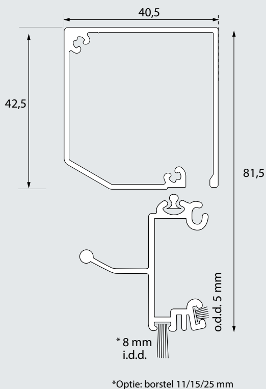
Doorsnede:
